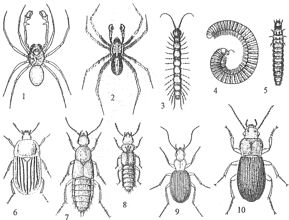
Obr. 91 Příklad zástupců epigeické fauny agroecozy; 1 – pavouk Erigone atra , 2 – pavouk Pardosa palustris , 3 – stonožka žltorohá ( Lamycetes fulvicornis ), 4 – mnohonozka Cylindroiulus teutonicus , 5 – páteříček sněhový ( Cantharis fusca ), 6 – mrchožrout Silpha tristis , 7 – drabčík Philonthus cognatus , 8 – drabčík Oxytelus rugosus , 9 – střevlík Anchomenus dorsalis , 10 – kvapník plstnatý ( Pseudoophonus rufipes ). Podle Tischlera, 1965.
