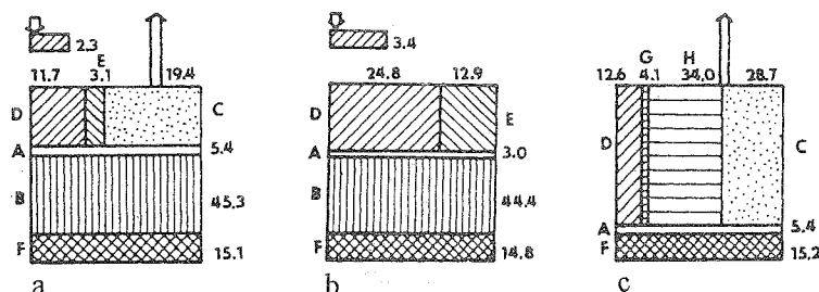
Obr. 88 Srovnání bilance hmoty produkčního lučního ekosystému (psárka luční, a), nevyužívaného společenstva zblochanu vodního (b) a pšenického pole (c, pšenice hnojená 120\text{ kg N} , 44\text{ kg P} a 150\text{ kg K}\cdot\text{ha}^{-1} ); šipky označují import a export hmoty; A – trvalá zásoba nadzemní biomasy (strniště), B – trvalá zásoba podzemní biomasy, C – hospodářský výnos, D – odumřelá nadzemní biomasa rozložená v létě, E – odumřelá nadzemní biomasa rozložená v zimě, F – podzemní roční produkce kořenové hmoty vstupující do dekompozice, G – listy pšenice, H – stéblo pšenice. Podle Rychnovské a Kruškové, z Petra a kol., 1980
