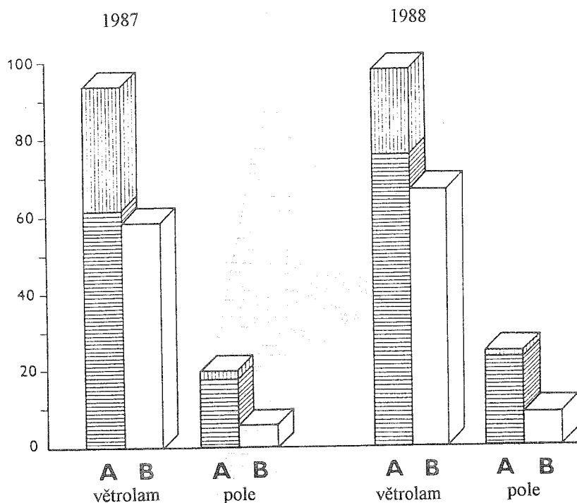
Obr. 92 Abundance (ex·m -2 ), biomasa (g·m -2 ) a rodové složení žížal ve větrolamu a sousedícím poli na jižní Moravě v letech 1987 a 1988; A – abundance, B – biomasa, horizontální šrafování – žížaly rodu Aporrectodea , vertikální šrafování – žížaly rodu Lumbricus a Octolasion . Podle Trnky a kol., 1990.
